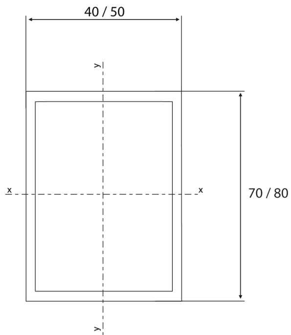
Stalen koker voor tentvloer
